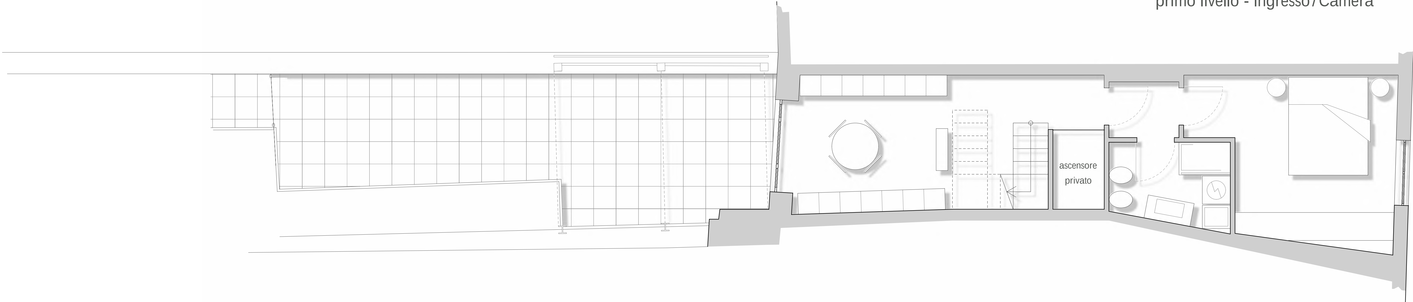
pianta primo livello - Ingresso / Camera
