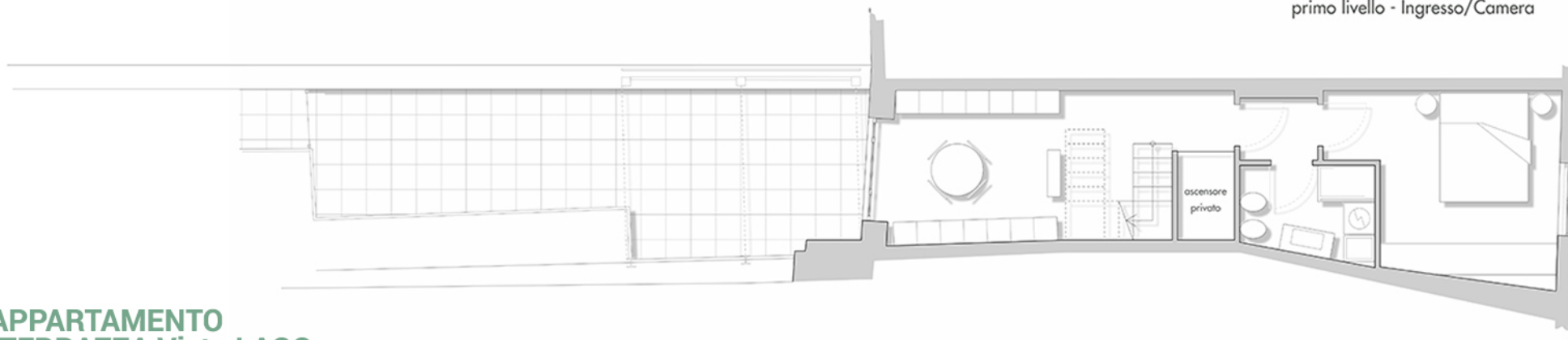
pianta primo livello - Ingresso/Camera
