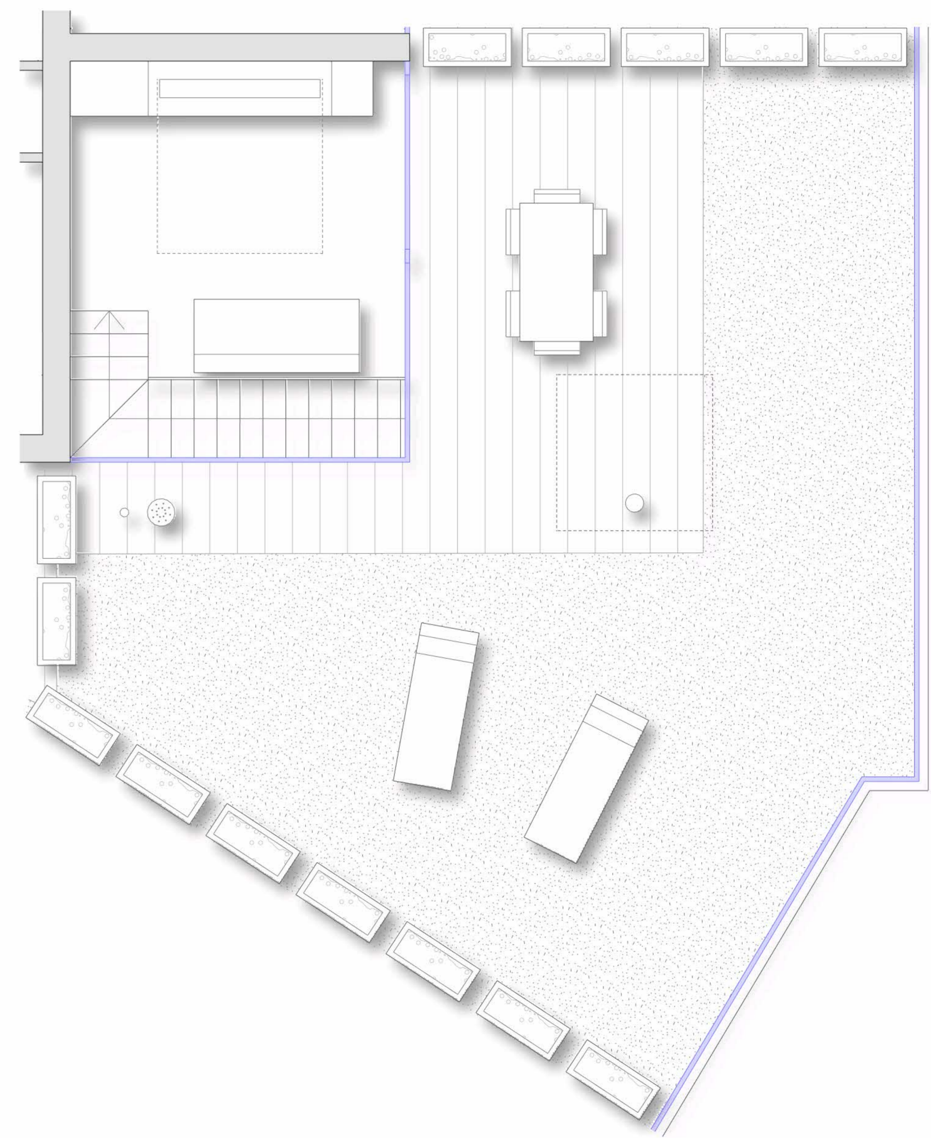
pianta piano terrazza
